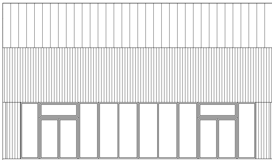
fasad C
