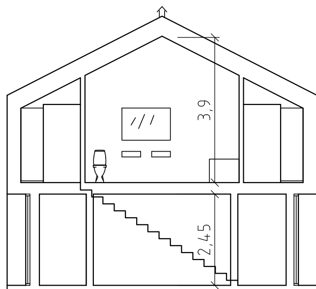
sektion
