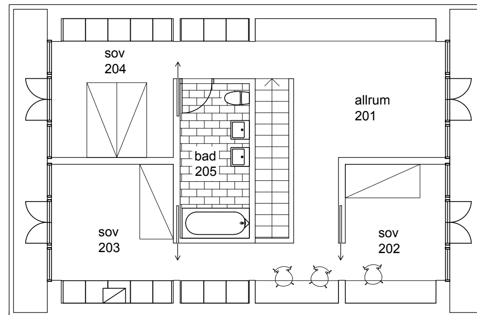
överplan
