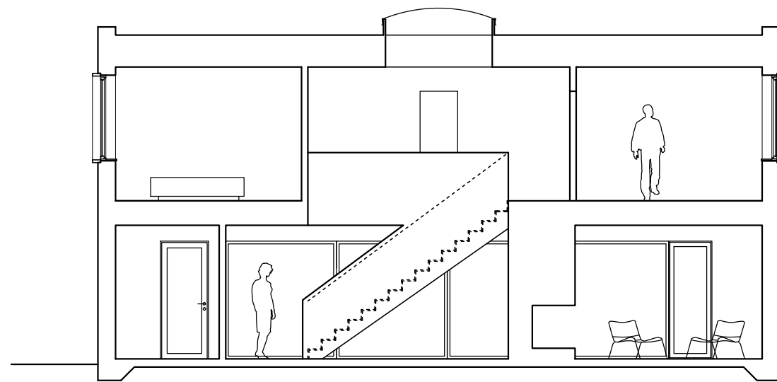
sektion A-A
