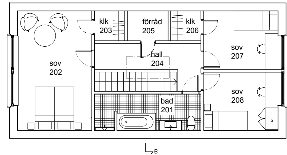
övreplan
