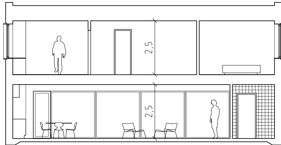
sektion A-A
