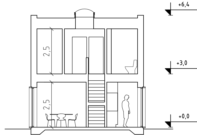
sektion B-B
