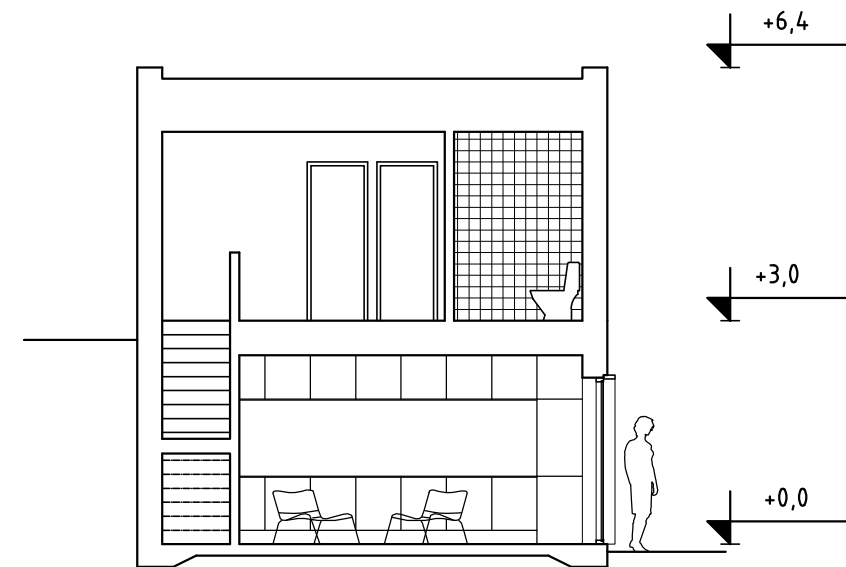
sektion B-B
