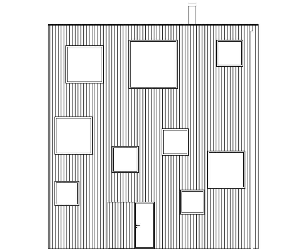
fasad D
