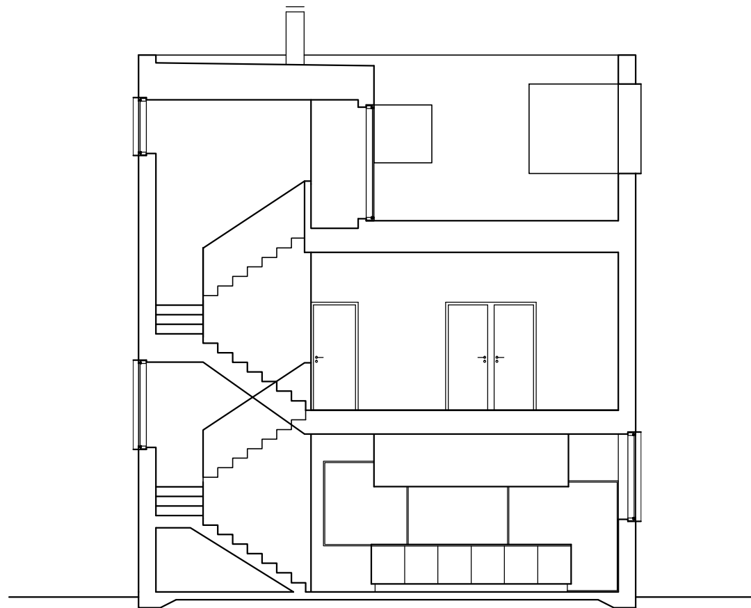
sektion A-A
