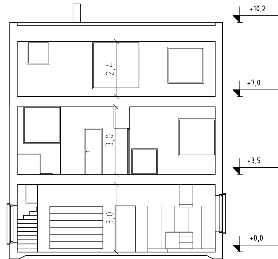
sektion C-C
