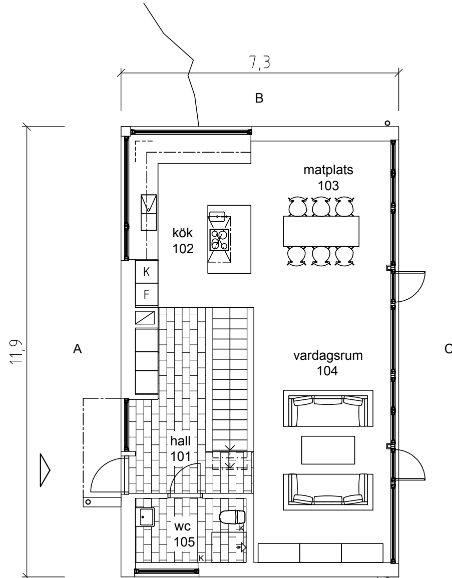
entréplan
