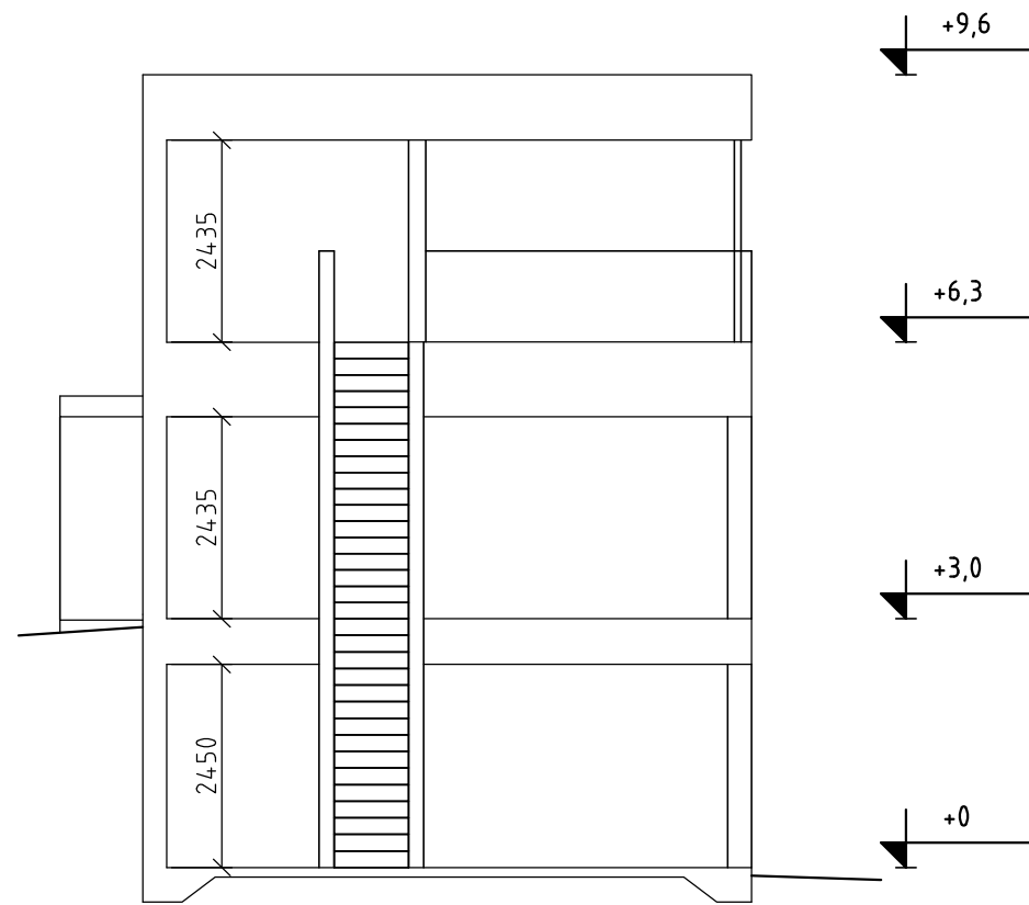
principsektion
