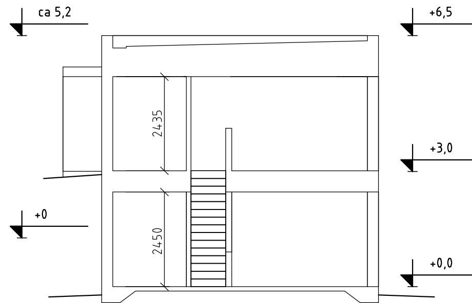
principlektion
