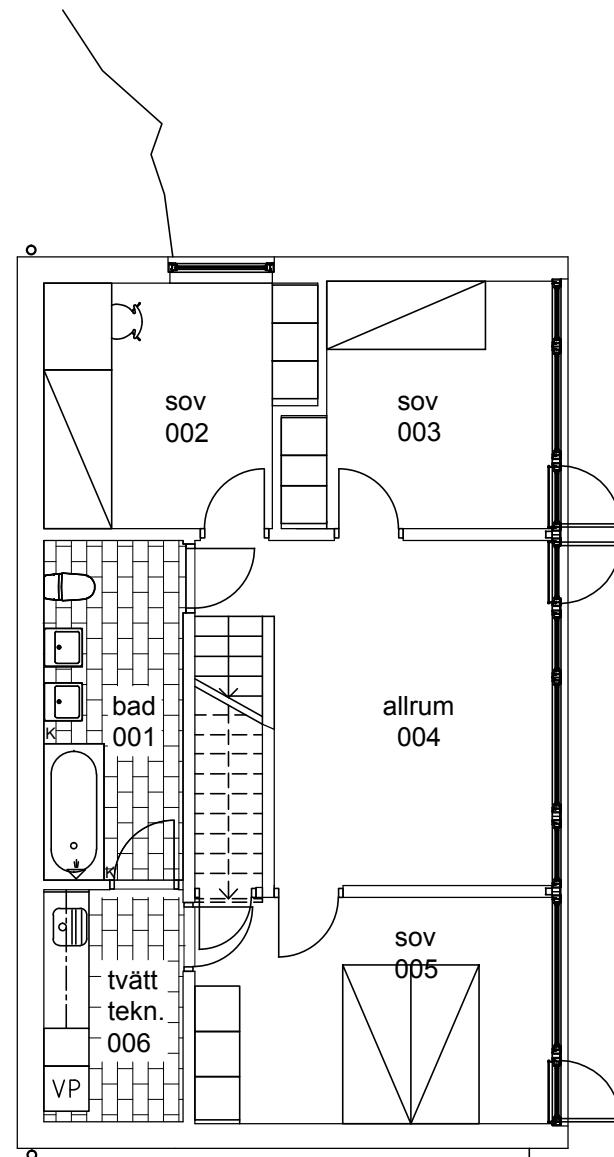
suterrängplan
