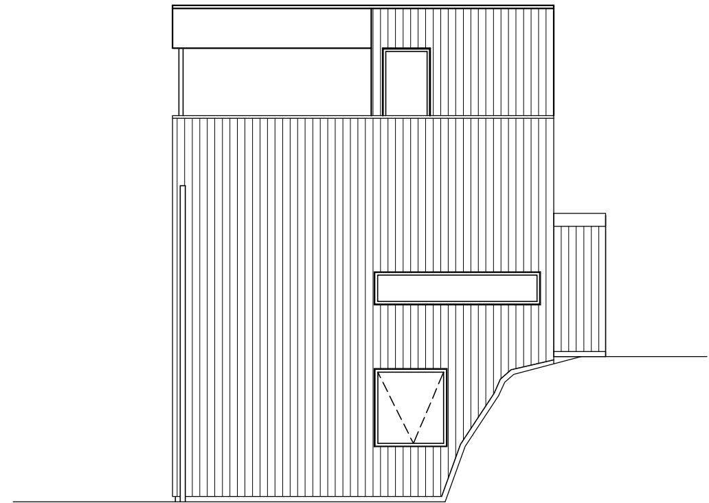
fasad B
